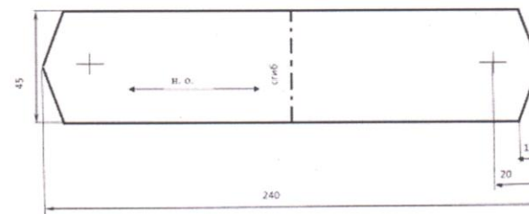
Чертеж 1. Основная деталь «Погон», 1 деталь со сгибом
