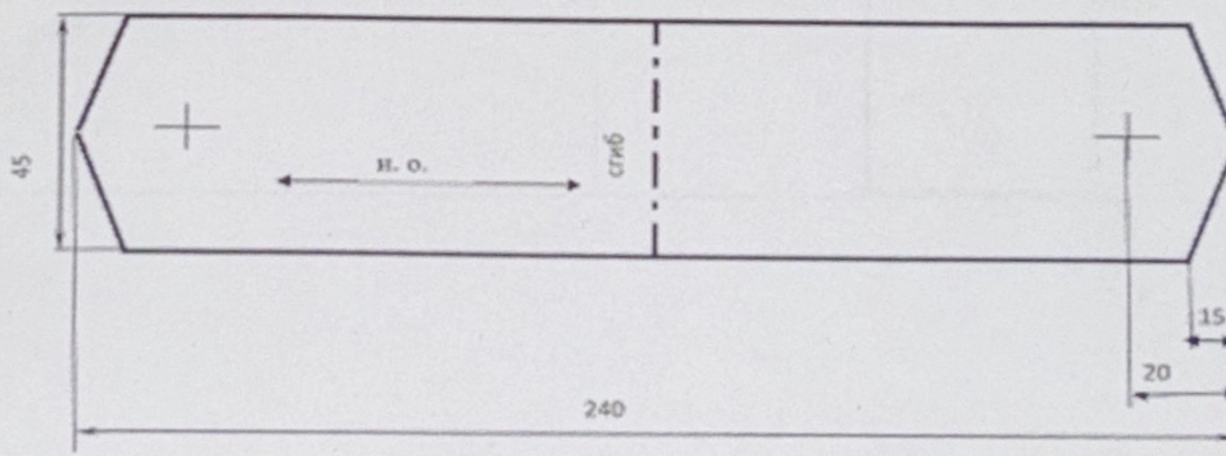
Чертеж 1. Основная деталь «Погон», 1 деталь со сгибом
