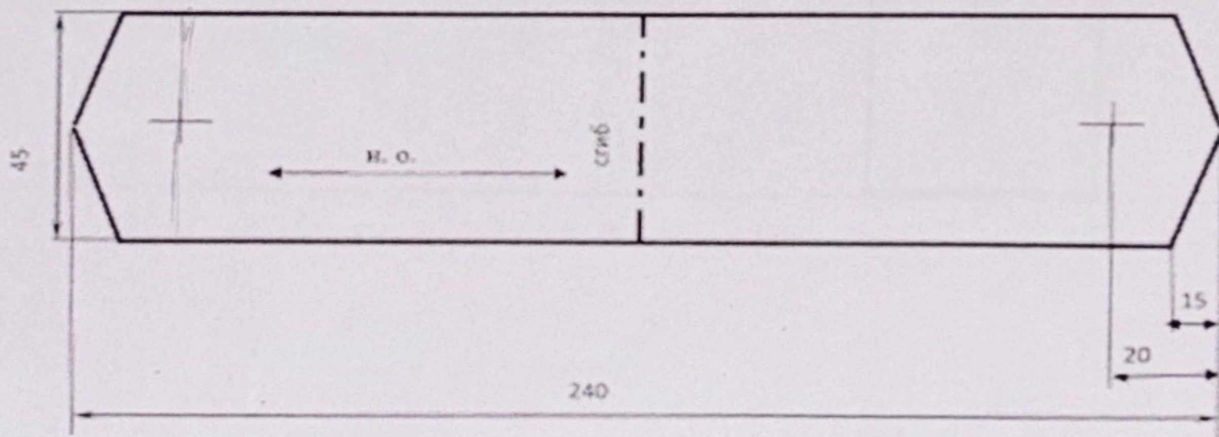
Чертеж 1. Основная деталь «Погон», 1 деталь со сгибом
