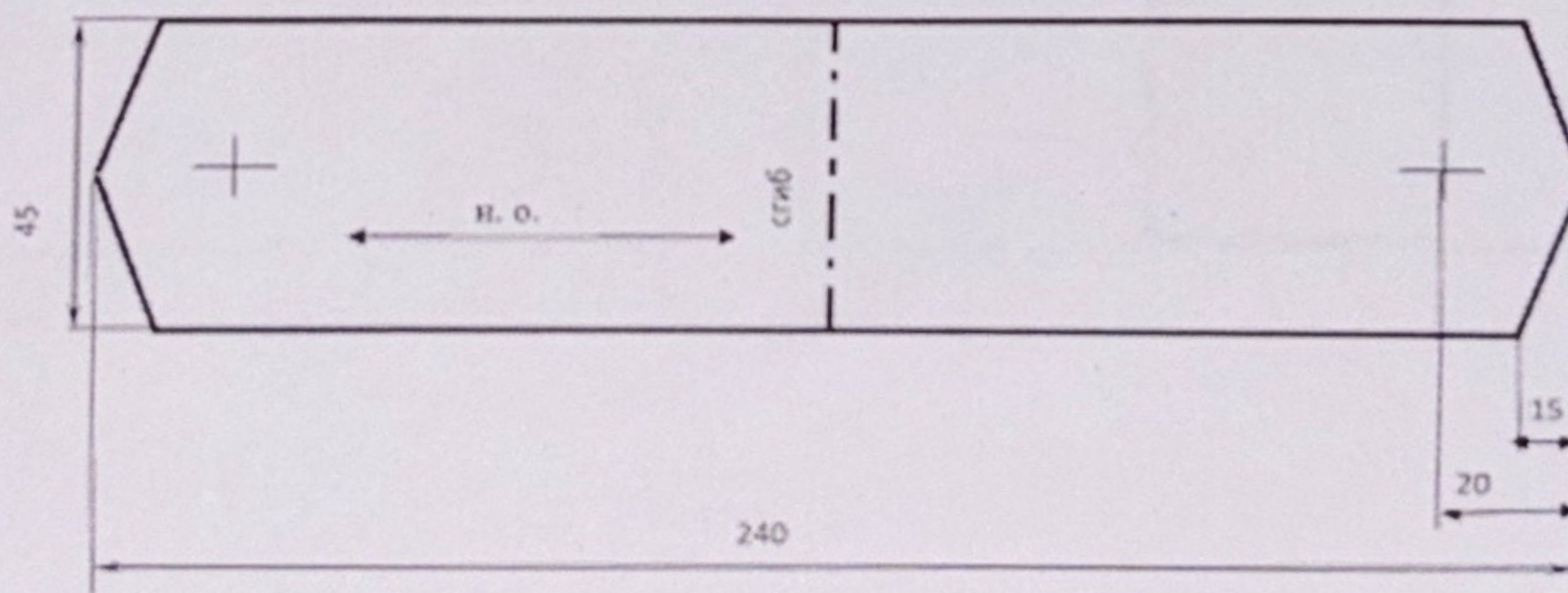
Чертеж 1. Основная деталь «Погон», 1 деталь со сгибом
