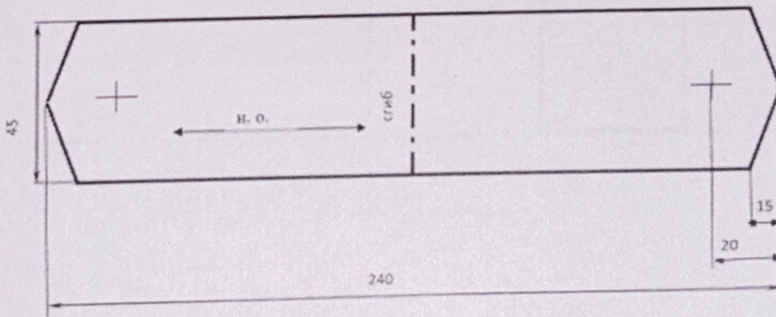
Чертеж 1. Основная деталь «Погон», 1 деталь со сгибом
