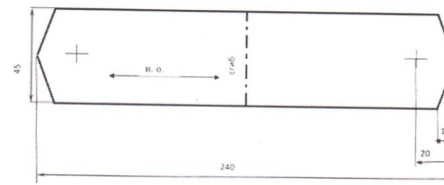
Чертеж 1. Основная деталь «Погон», 1 деталь со сгибом
